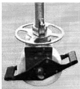
Kółko jezdne zablokowane
